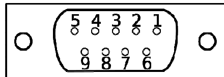
Draufsicht D-Sub Stecker am Kabel (female)
