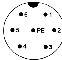
Draufsicht Rundstecker (male) Anschluss innen an die USB-Box oder an das Wiegeterminal
