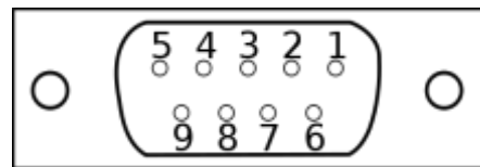
Draufsicht D-Sub Stecker am Kabel (female)
