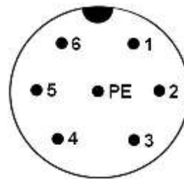
Draufsicht Rundstecker (male) Anschluss innen an die USB-Box oder an das Wiegeterminal
