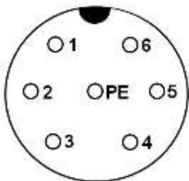
Draufsicht Rundstecker (female) Anschluss außen an die Wiegeelektronikbox
