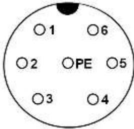
Draufsicht Rundstecker am Kabel (female)
