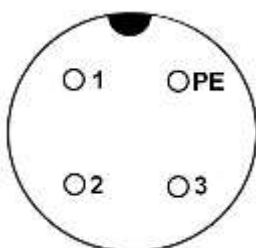
Draufsicht Rundstecker am Kabel (female)
